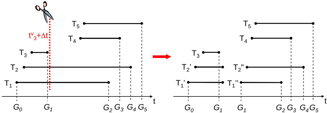
4-2. ábra: Egy korai tranzakciólezárást tartalmazó szerkesztési szakasz tranzakcióinak beosztása egy T_1^S = T_1', T_2', T_3 és egy T_2^S = T_1'', T_2'', T_4, T_5 tranzakciósorra.
