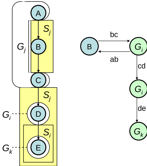
5-1. ábra: Példa olyan szerkesztési esetre, melyben az A2 és A3 integrációjaként kapott A4 azoknál jobb eredményt ad. A bal oldalon a gráf, mellette pedig az ebből A3 által készített szomszédossági gráf látható.
