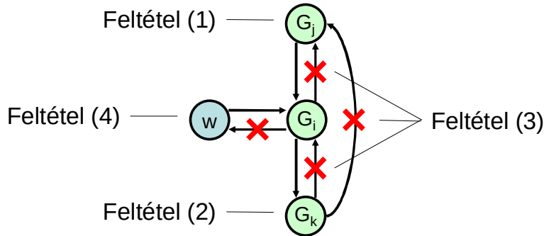
4-9. ábra: Feltételrendszer, amely megadja, hogy milyen gráfstruktúra és tranzakcióesetén lehet A3 \wedge A2 .
