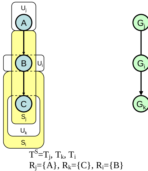
4-10. ábra: Egy minimális G, T^S pár, amelyre A3 \preceq A2 . Bal oldalon a gráf látható A2 zárjaival, jobb oldalon pedig az A3 által készített szomszédossági gráf.
