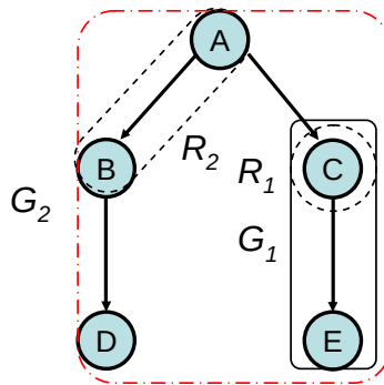
3-7. ábra: Példa olyan kollaboratív szerkesztési esetre melyet az A1 algoritmus tilt, holott a felhasználók munkája különböző gráfreszeket érint.
