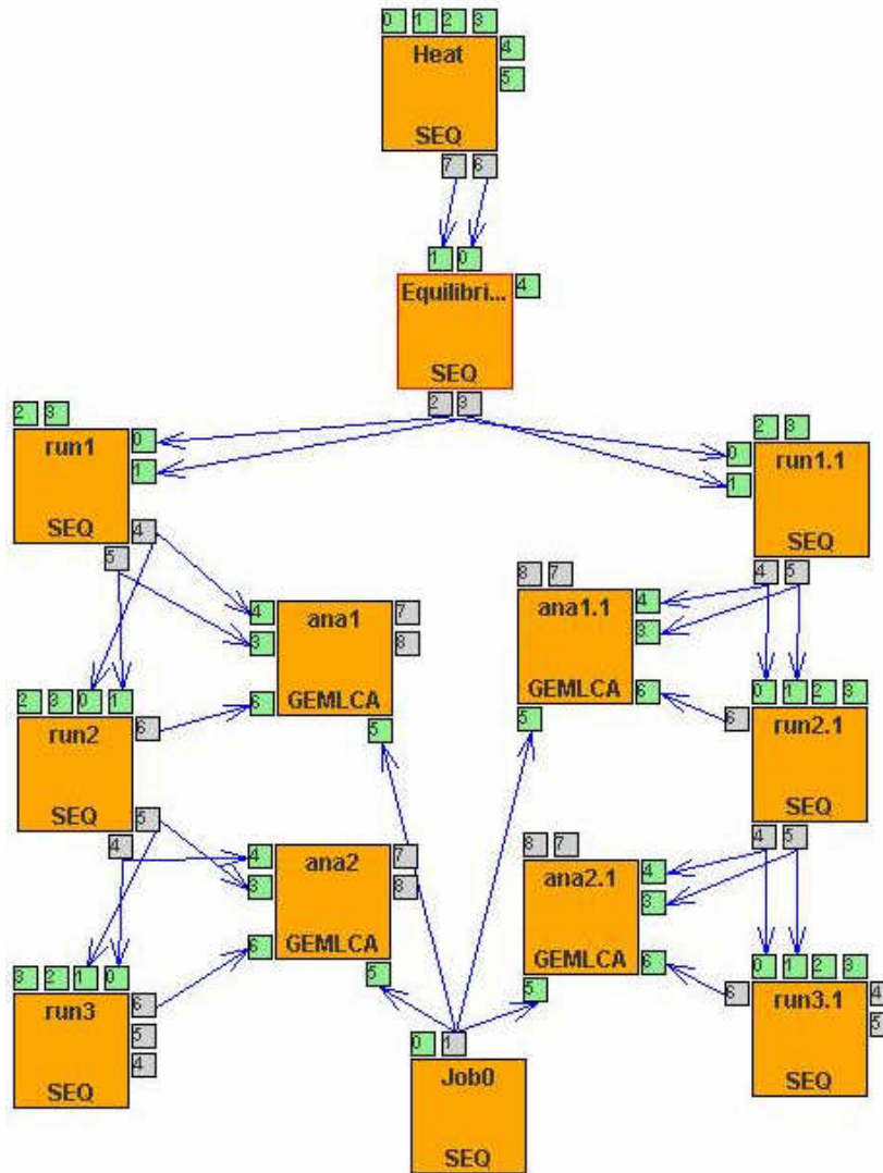
5-12. ábra: CHARMM workflow WS-PGRADE környezetben
