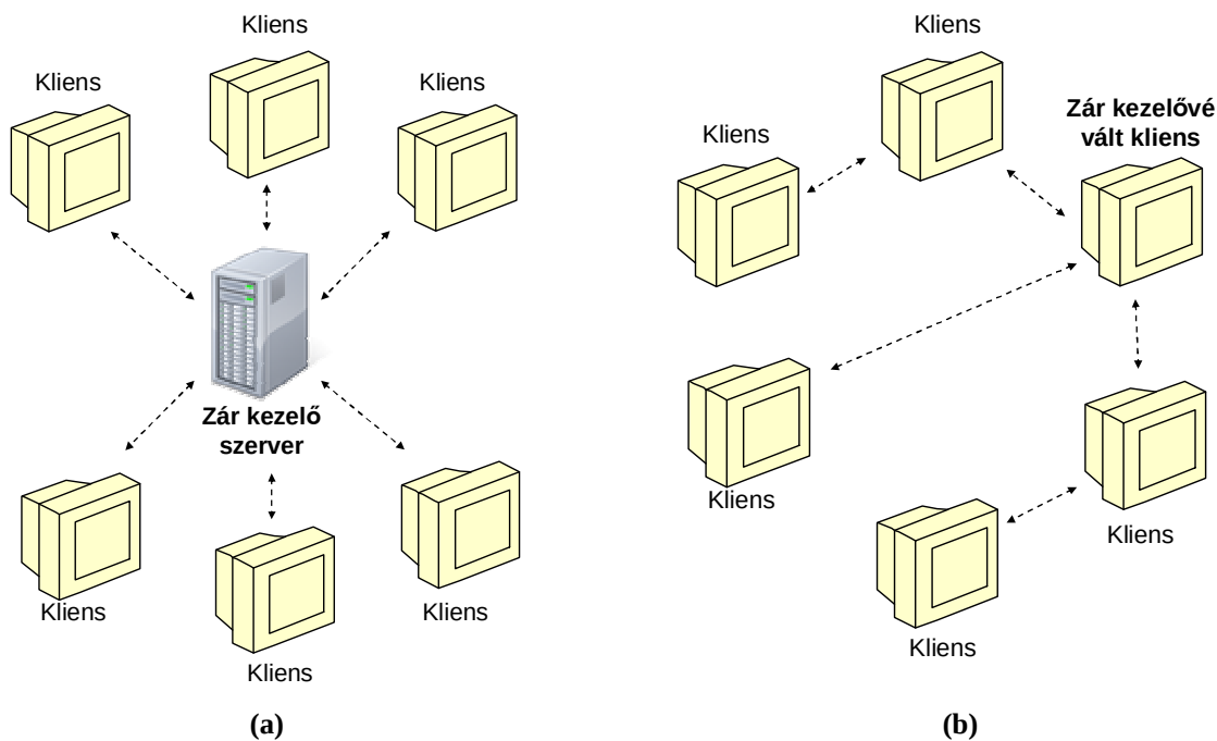
2-5. ábra: Zár kezelés (a) dedikált szerver és (b) menedzserré váló kliens gép segítségével.
