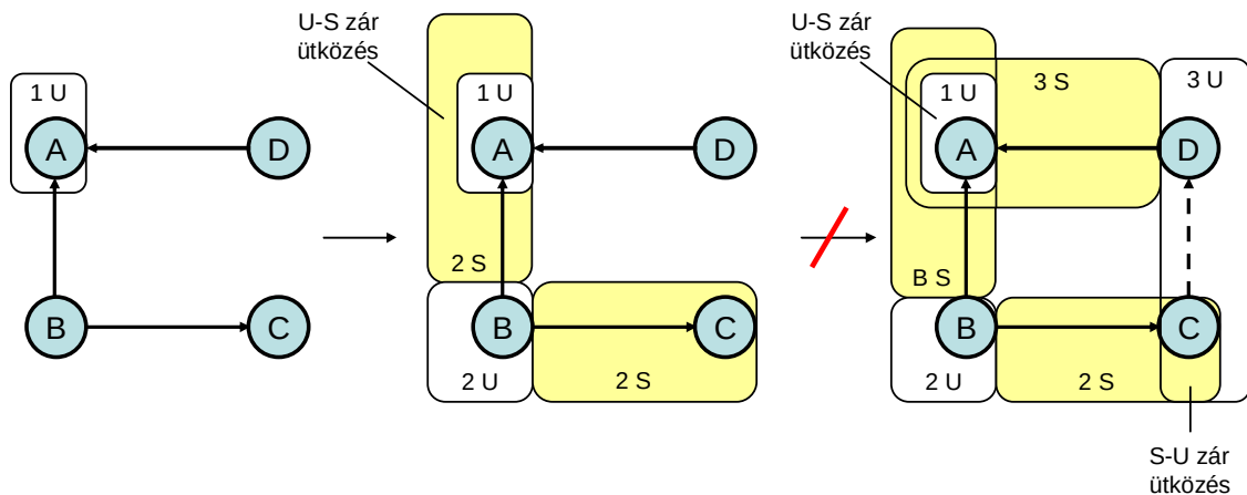
4-7. ábra: A2 algoritmus zárjai egy A3 \nless A2 esetre.
