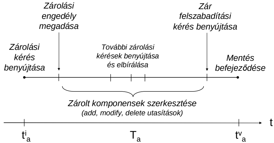
2-6. ábra: Egy T_a workflow szerkesztési tranzakció teljes életciklusa.
