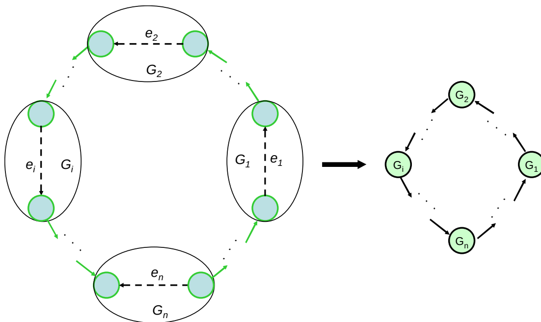
3-14 ábra: Gráfok körmentességének biztosítása szomszédossági gráf segítségével.
