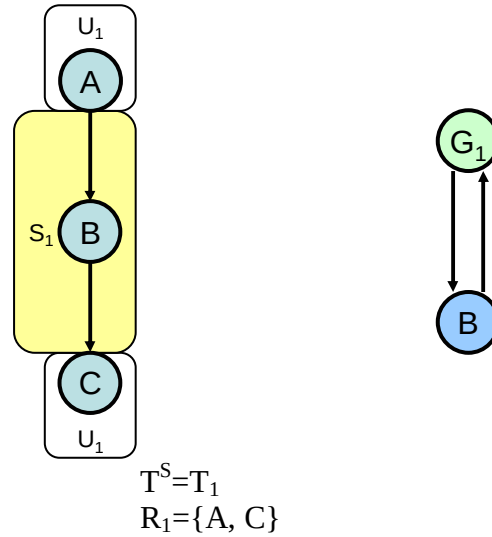
4-17. ábra: Egy olyan minimális gráf-tranzakciósor pár, amelyre A2 \preceq A3 . Bal oldalon a gráf látható A2 zárjaival, jobb oldalon pedig ugyanerre az esetre az A3 által készített szomszédossági gráf.
