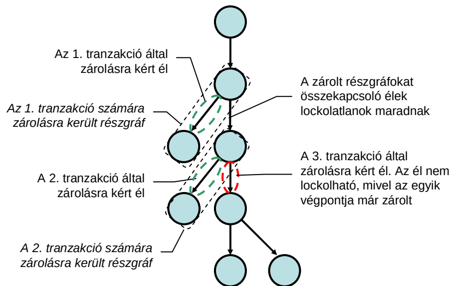
3-2. ábra: Szabad élek elleni védelmet biztosító protokoll használat közben.
