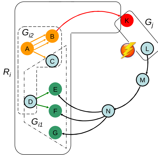
5-13. ábra: A5 által tiltott kérés helyett felajánlható egy alternatív zárolható részgráf. A súlyozási függvénytől függően vagy a G_{i1} , vagy a G_{i2} részgráf ajánlható fel az R_i zárolási kérést beküldő felhasználó számára.
