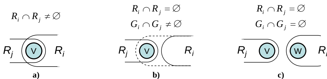
5-4. ábra: A4 által tiltott, konzisztenciát nem sértő tranzakció kategorizálása. (Két tranzakció gráfot érintő módosításának átfedési lehetőségei.)
