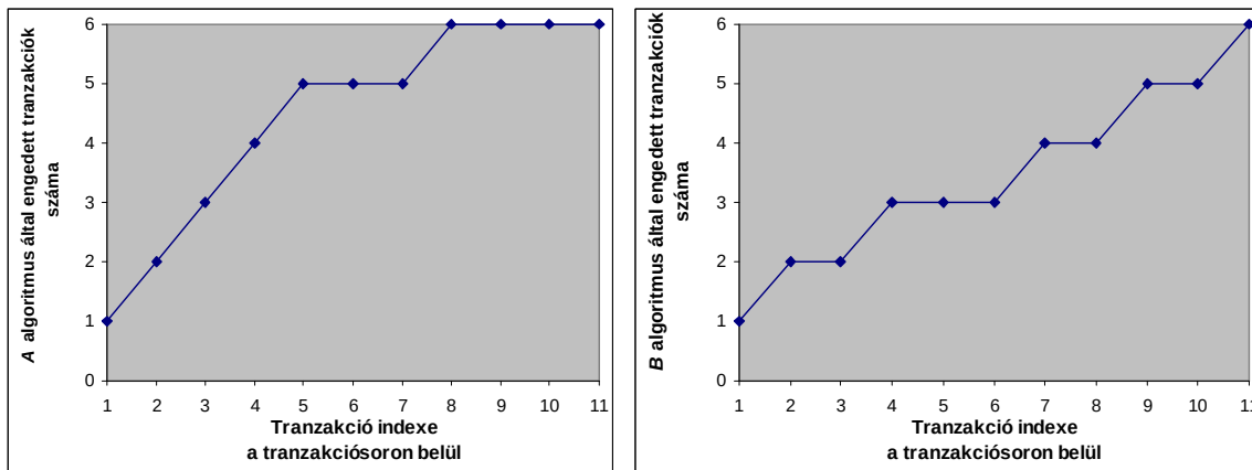
4-4. ábra: Igazságossági reláció demonstrálása függvénnyel. Az A és B algoritmusok ugyanolyan jók. A kettő közül A az igazságosabb. Ez a függvényekből onnan látszik, hogy A függvénye éri el hamarabb a maximumát.
