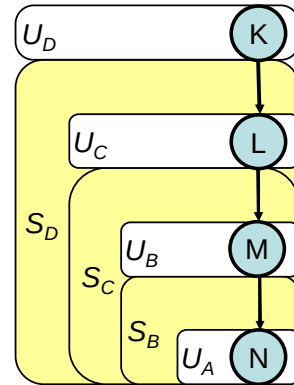
3-12. ábra: Az S lock-ok újragenerálását a tranzakciók indulási sorrendjének megfelelően kell végrehajtani, különben már futó tranzakciók eredményezhetnek tiltott ütközést.
