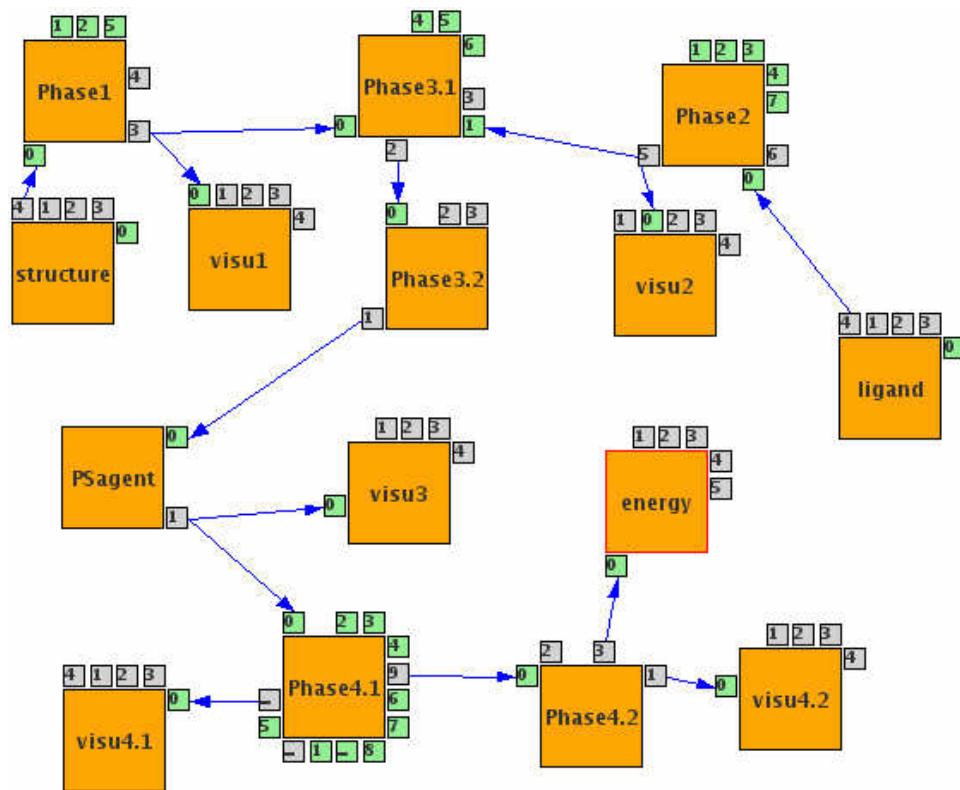
4-21. ábra: Proteine molecule workflow WS-PGRADE környezetben
